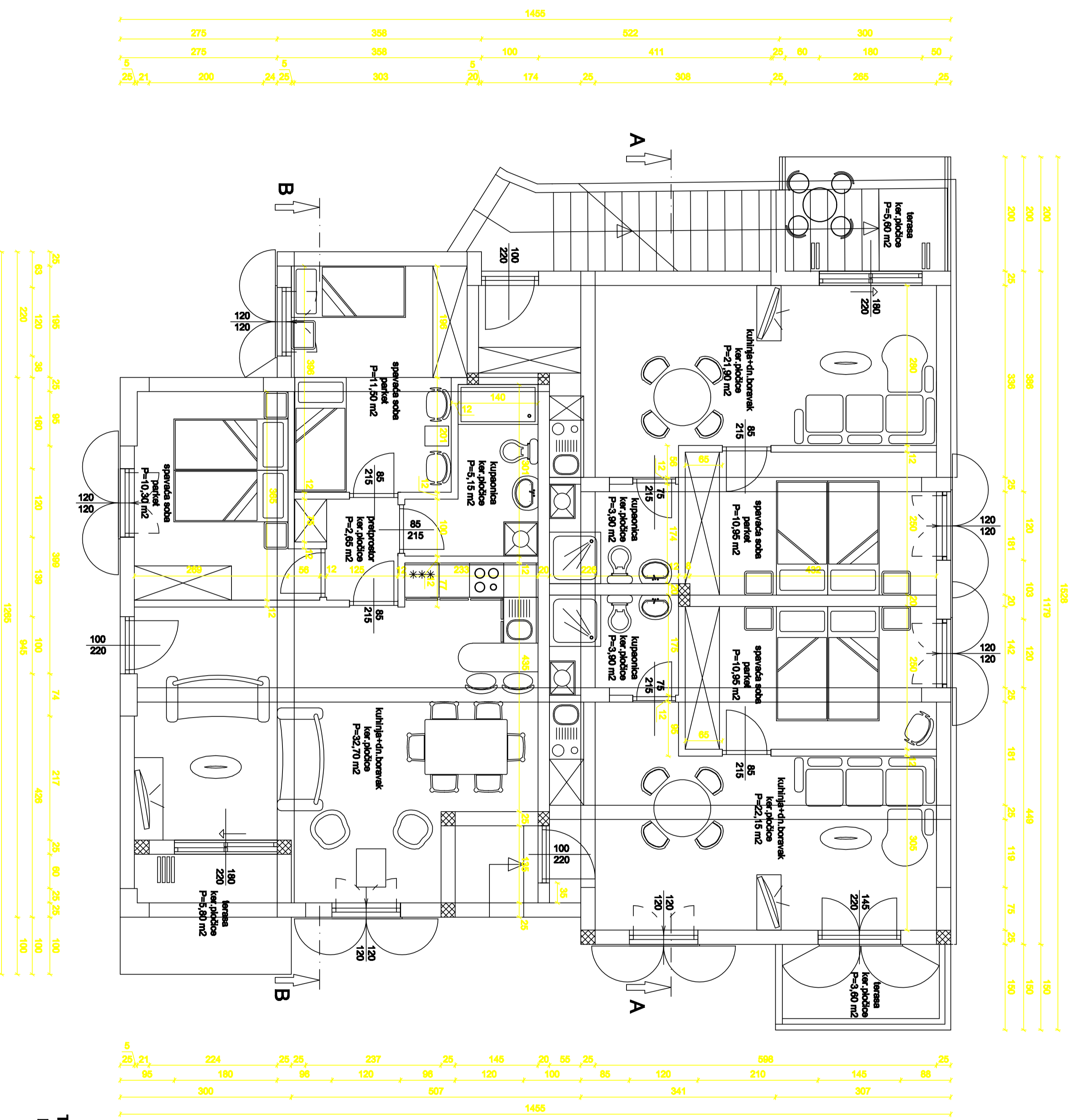
TLOCRT PRIZEMLJA projektirano stanje M 1:50
