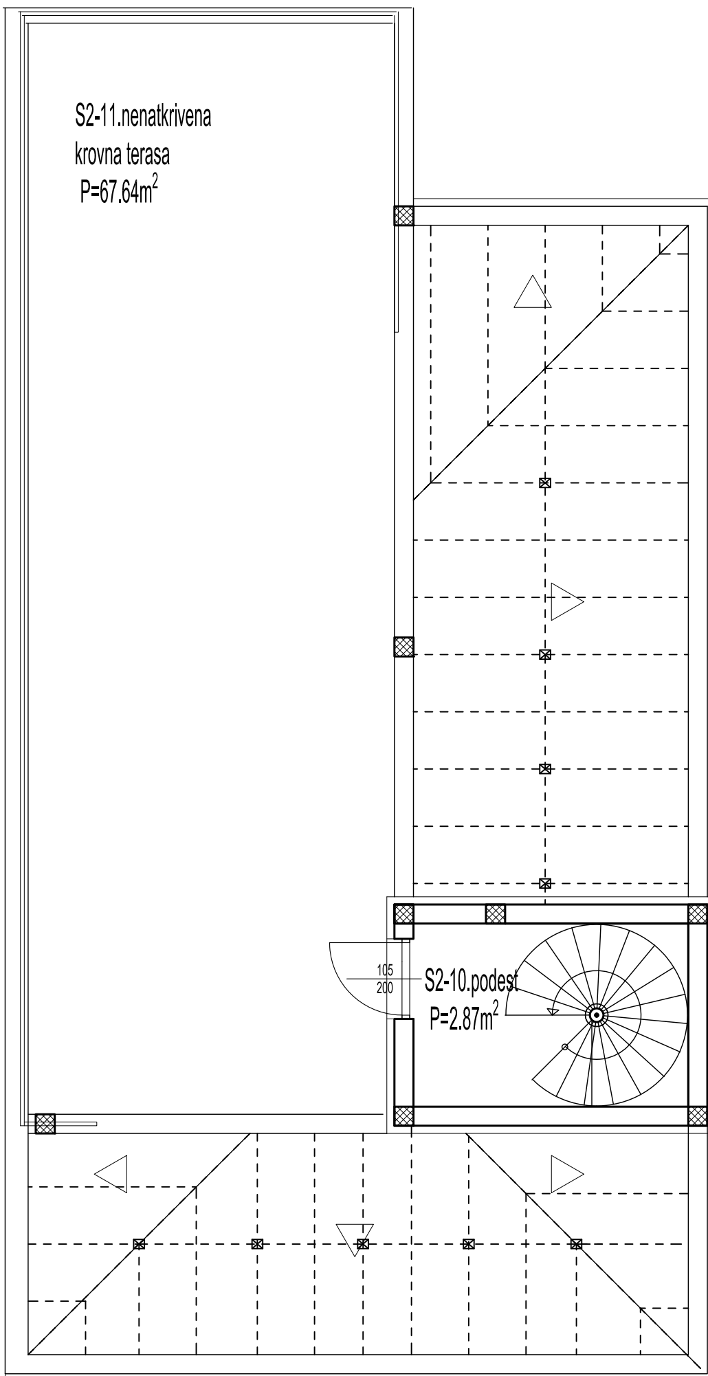
TLOCRT KROVNE TERASE
