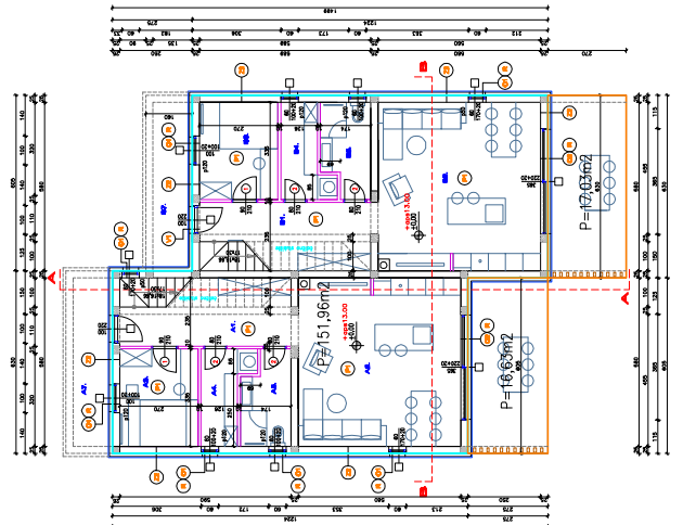
TLOCRT PRIZEMLJA M 1 : 100
