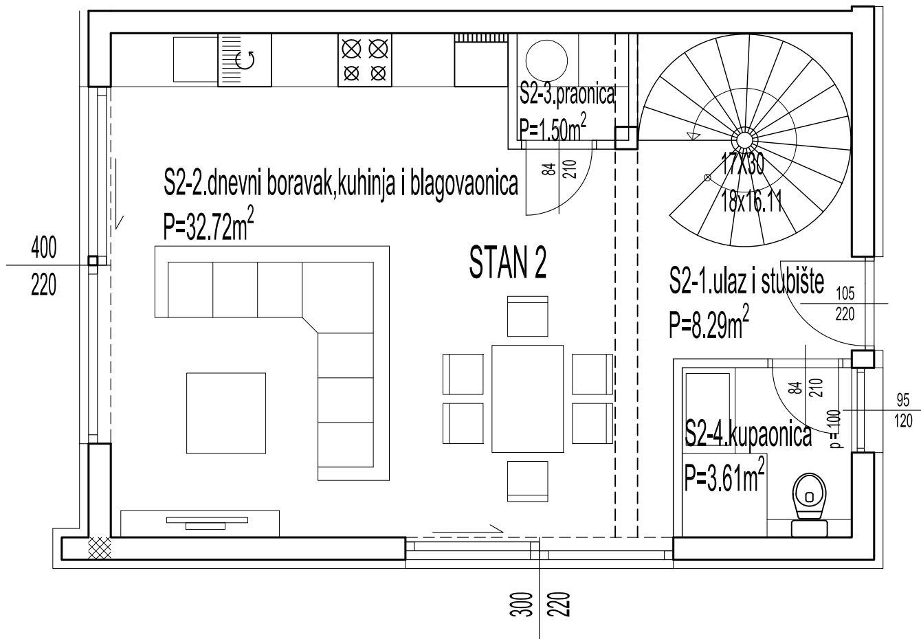
TLOCRT PRIZEMLJA
