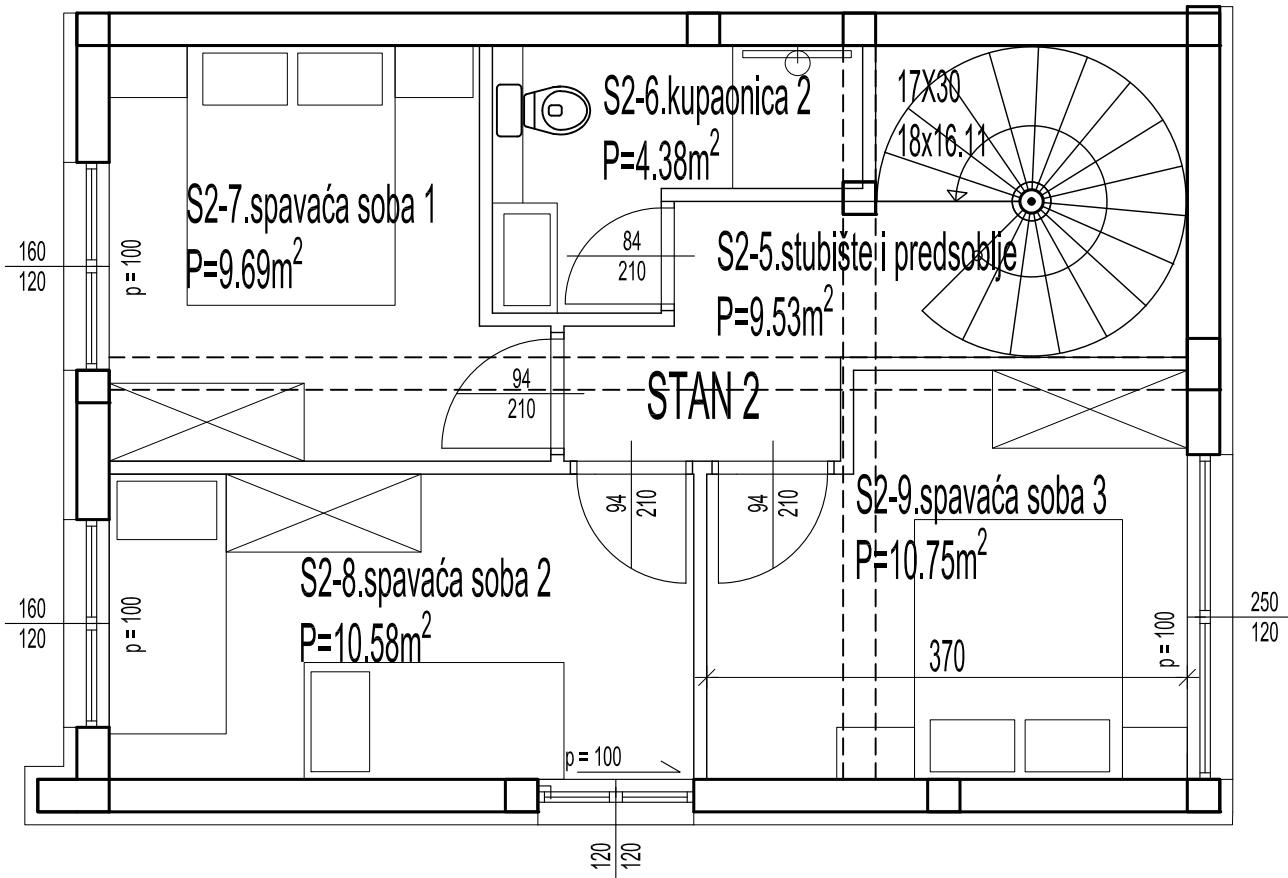
TLOCRT KATA
