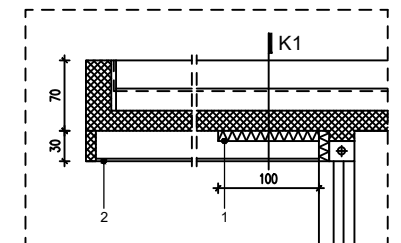
DETALJ 2
