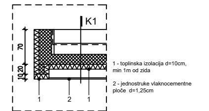
DETALJ 1
